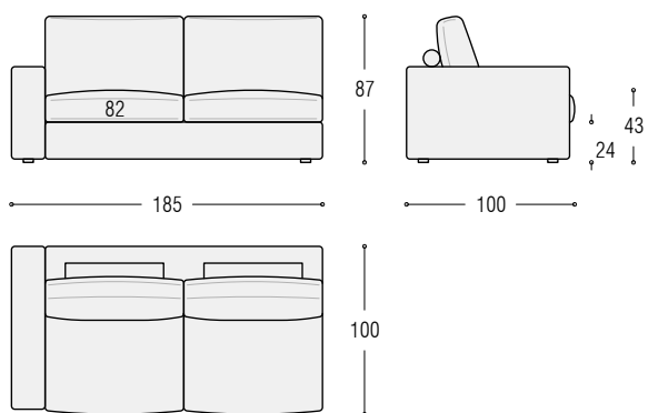
Element cm 185 left
